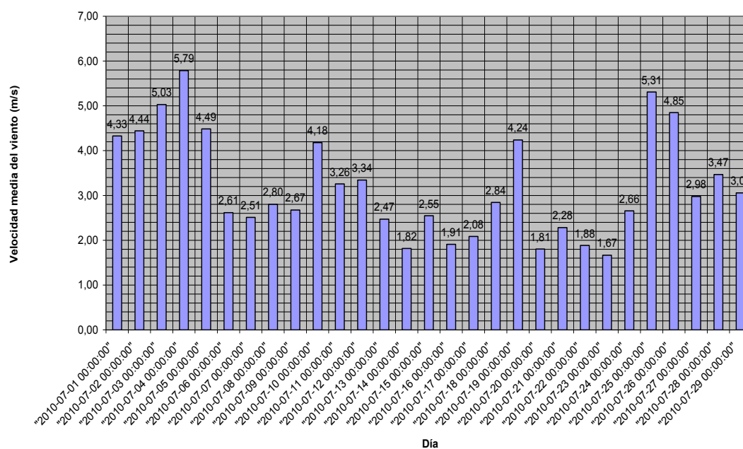
PERFIL DE VIENTOS DE JULIO 2010 (HUERTO EXTREMADURA)
