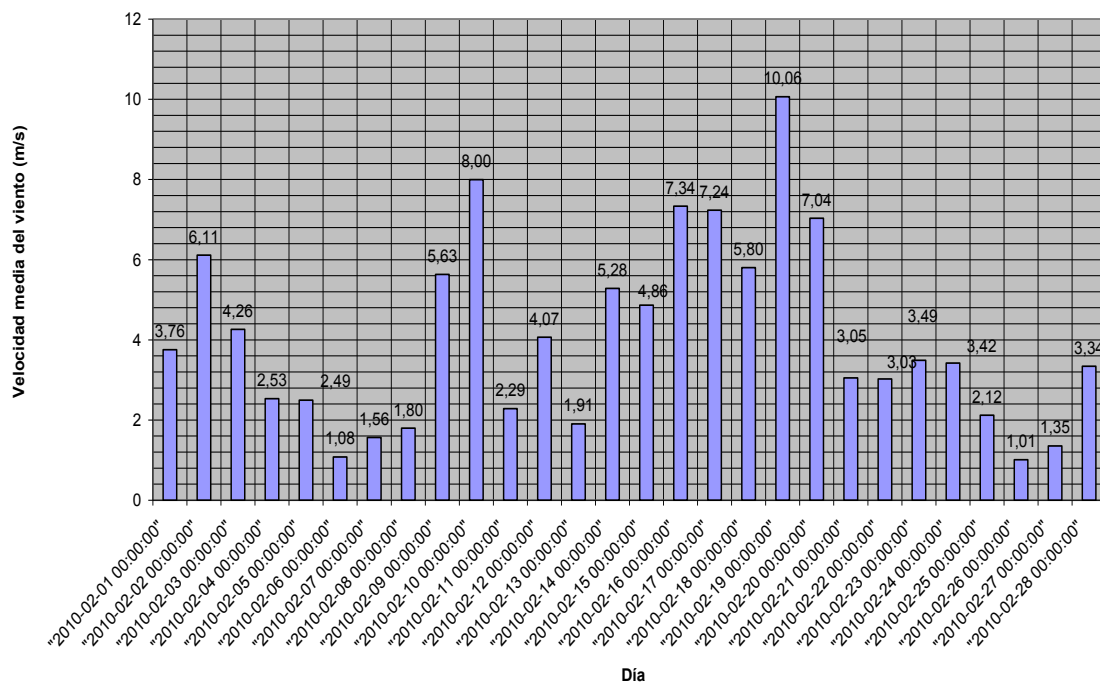
PERFIL VIENTOS FEBRERO 2010 (HUERTO DE EXTREMADURA)
