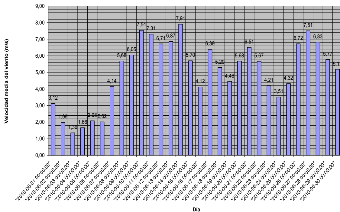
PERFIL DE VIENTOS JUNIO 2010 (HUERTO EXTREMADURA)
