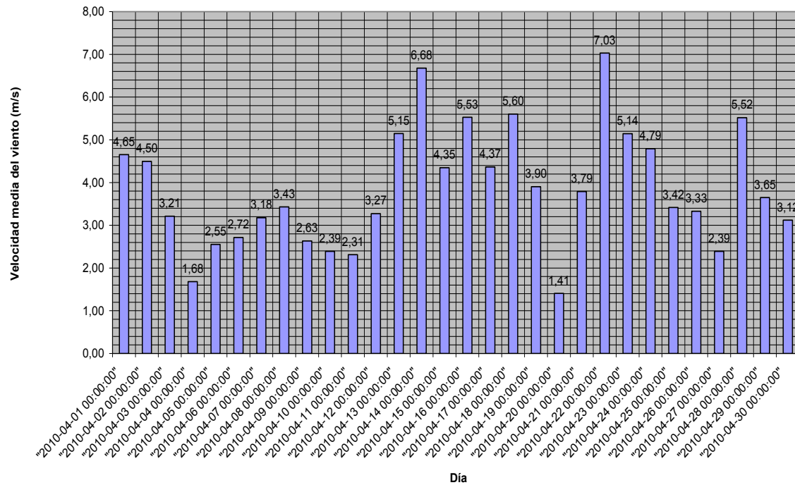
PERFIL VIENTOS ABRIL 2010 (HUERTO DE EXTREMADURA)
