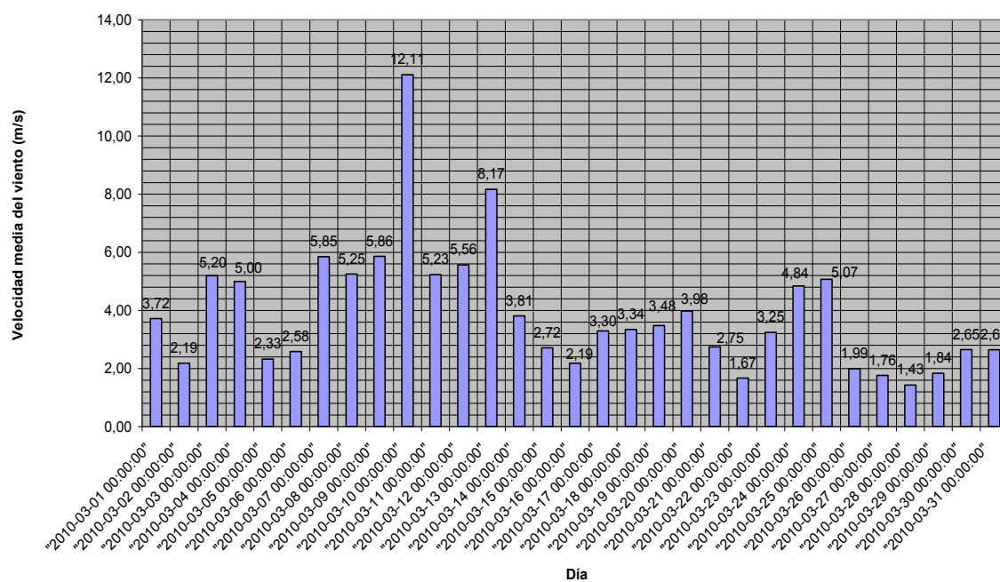
PERFIL VIENTOS MARZO 2010 (HUERTO EXTREMADURA)
