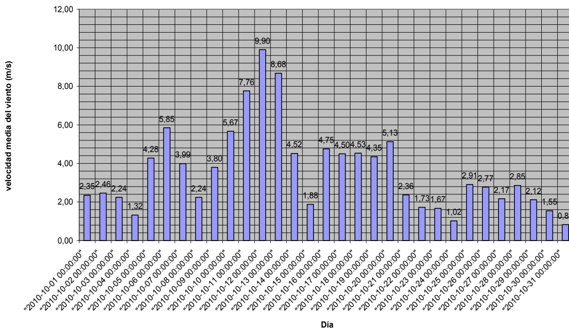
PERFIL DE VIENTOS OCTUBRE 2010 (HUERTO EXTREMADURA)
