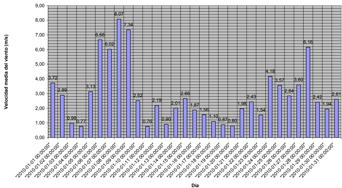
PERFIL VIENTOS ENERO 2010 (HUERTO EXTREMADURA)
