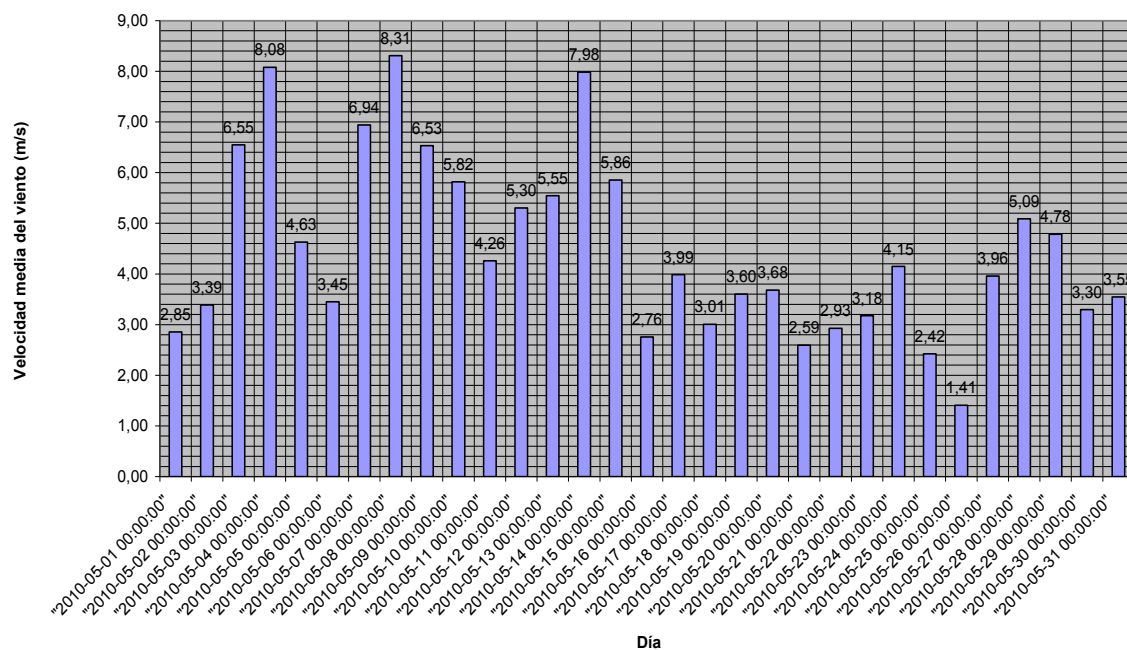
PERFIL DE VIENTOS MAYO 2010 (HUERTO EXTREMADURA)
