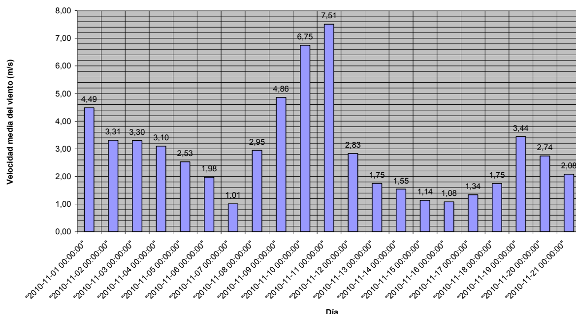
PERFIL DE VIENTOS NOVIEMBRE 2010 (HUERTO EXTREMADURA)
