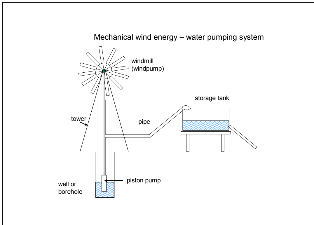
Figura 20. Esquema básico de funcionamiento del molino eólico para bombeo de agua. El tanque permite dar la presión necesaria para el sistema de riego.
